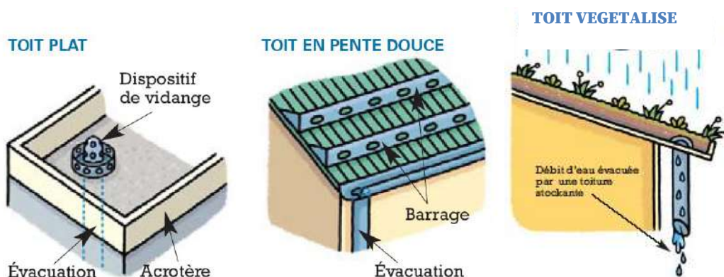
PRINCIPES DES TOITURES STOCKANTES (A GAUCHE ET AU CENTRE) ET VEGÉTALISÉE (A DROITE)
