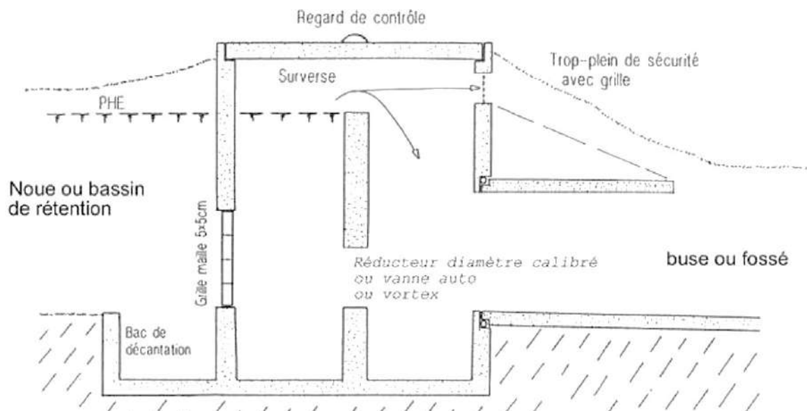
PETIT OUVRAGE EN BÉTON AVEC ORIFICE ET SURVERSE INTÉRIEURE
