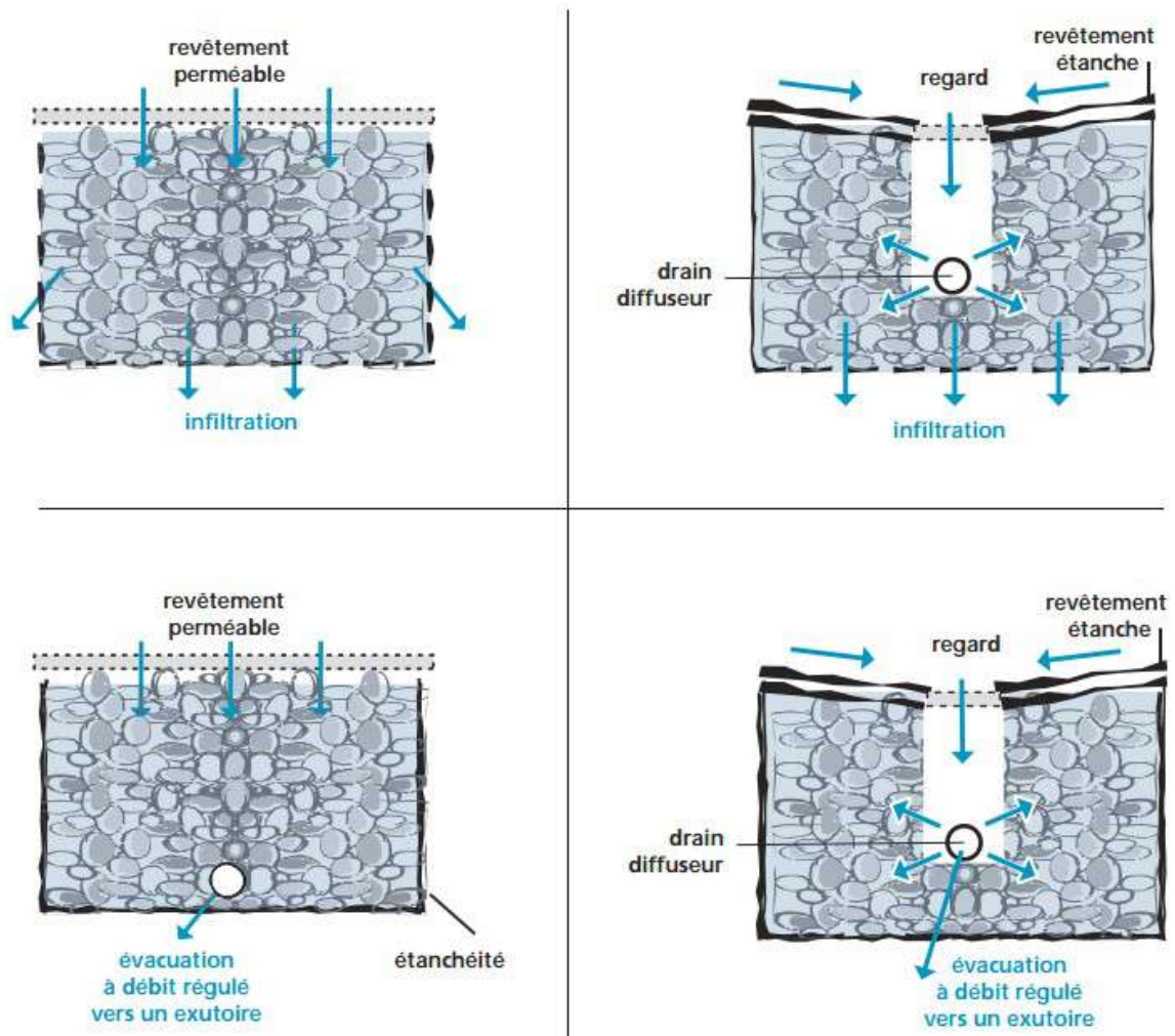
DIFFÉRENTS TYPES DE STRUCTURES RÉSÉROIR (SOURCE : GRAIE)
